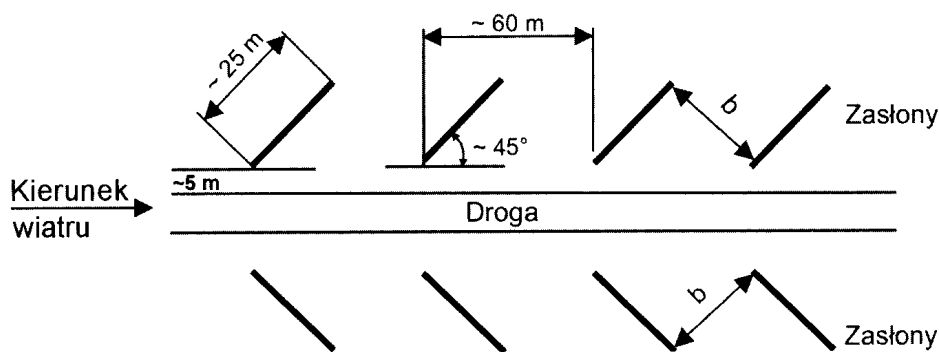
Rys. 7. Ustawianie zasłony przy kierunku wiatru pokrywającym się z kierunkiem drogi (wg [2])
